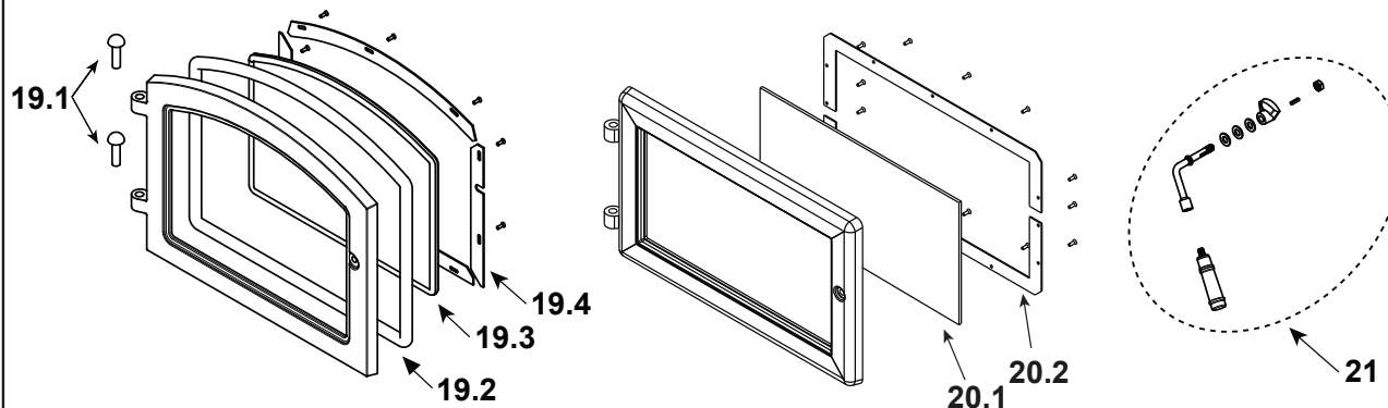
#19 Arch Door Assembly
