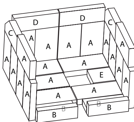
Positionnement des briques
