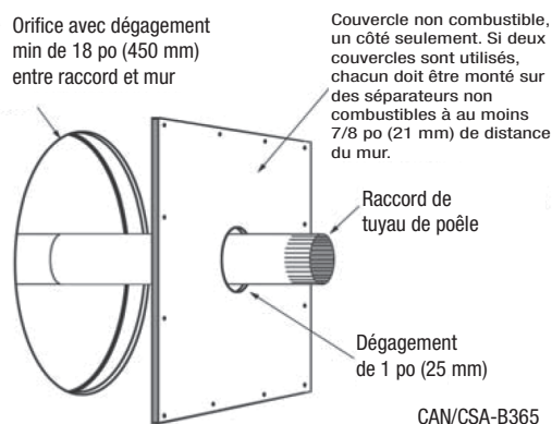
Figure 4 SEUL PASSE-MUR APPROUVÉ AU CANADA
